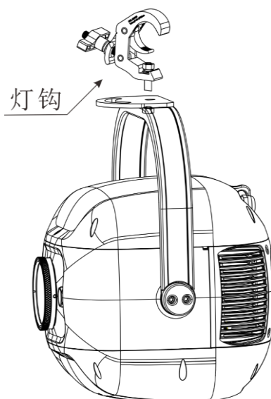
吊挂放置图
