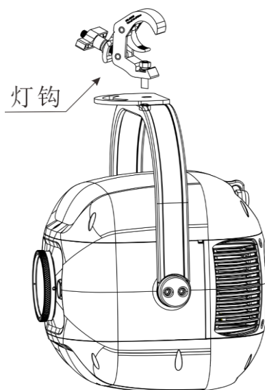
吊挂放置图
